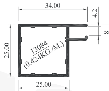
13084 (0.424Kg./M.) KT - One Side
